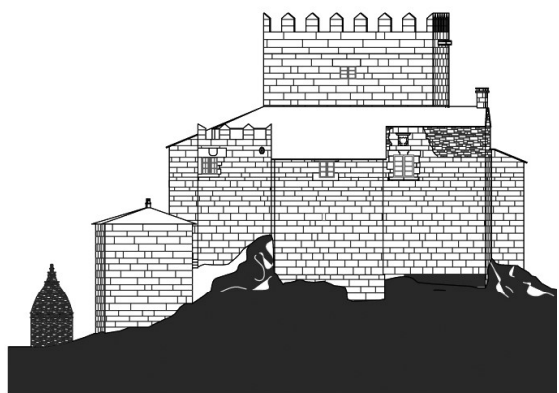
Alzado norte da Fortaleza de San Paio de Narla. Ano 2011
