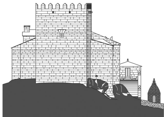
Alzado sur da Fortaleza de San Paio de Narla. Ano 2011
