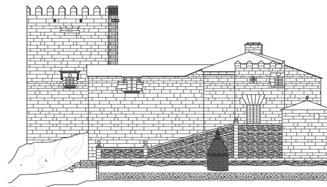
Alzado este da Fortaleza de San Paio de Narla. Ano 2011
