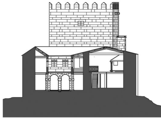
Alzado sur da Fortaleza de San Paio de Narla. Ano 2011
