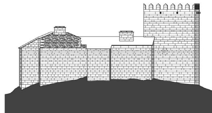
Alzado oeste da Fortaleza de San Paio de Narla. Ano 2011
